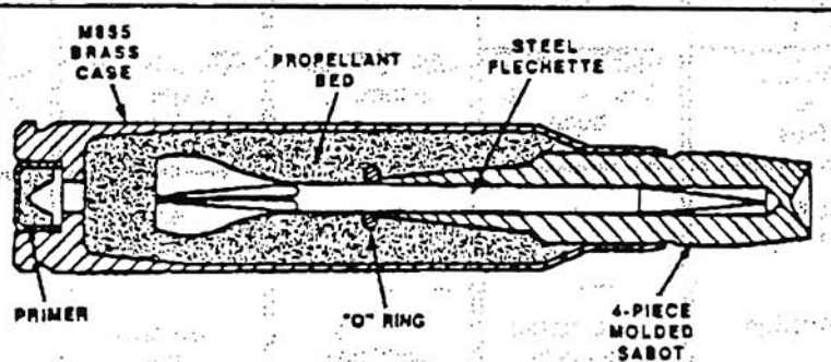
AAI FLECHETTE AMMUNITION
